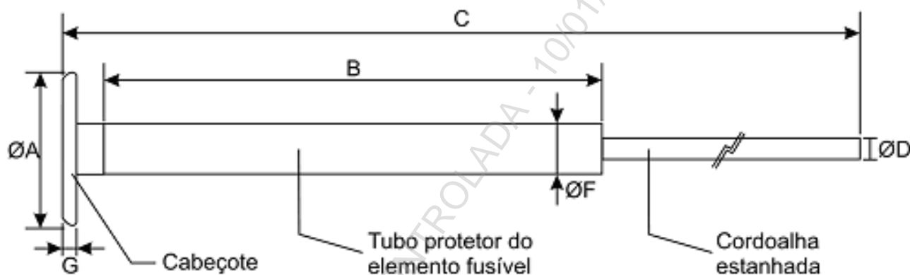
Figura 1 - Elo Fusível com Botão Fixo
